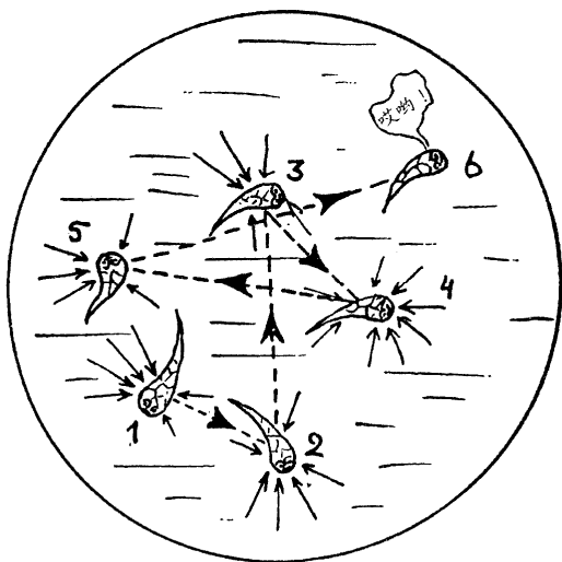
图 77 一个细菌被周围分子推来揉去而连续换了六个位置
