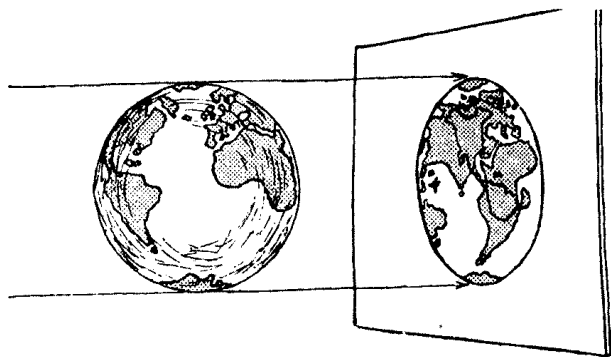
图 27 圆球的平面投影
