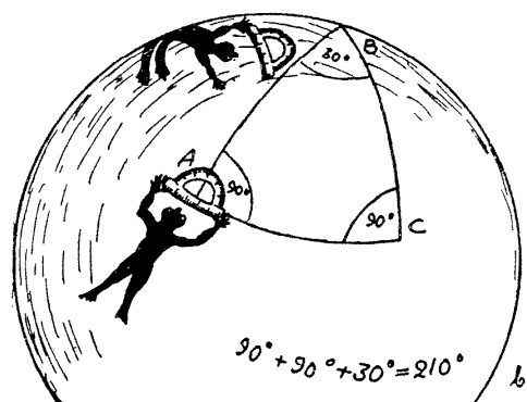
图 39 “平面世界”和“曲面世界”上的扁片科学家们在检验三角形的内角和是否符合欧几里得定理
