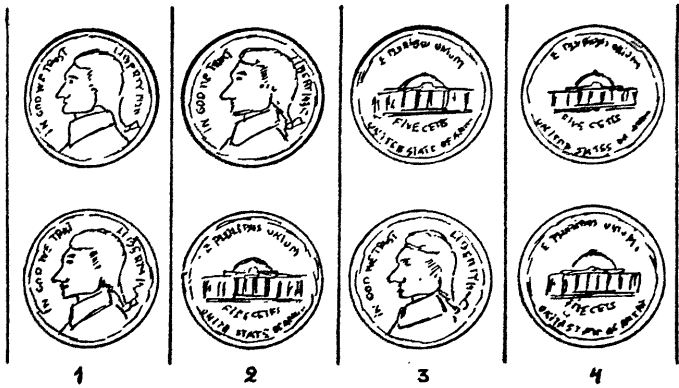
图 83 掷两枚硬币的四种可能性
