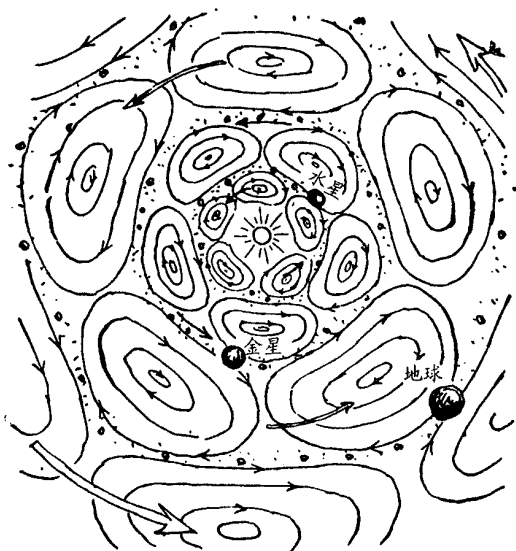
图 120 在早期的太阳包层中微尘的通道
