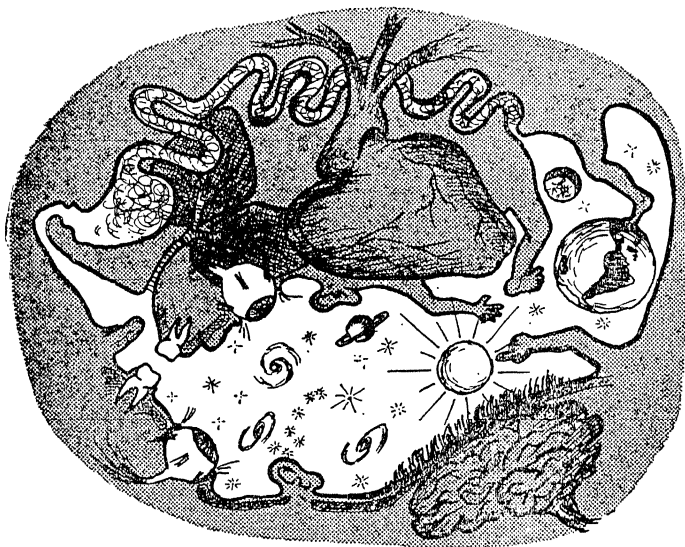
图 20 翻过来的宇宙。这幅超现实的图画所画的是一个人在地球表面上走，并抬头看着星星。这幅画是用图 19 所示的方法进行拓扑学变换的。地球、太阳和星星都被挤到了人体内的一个狭窄的环形通道里，它们的四周是人体的内部器官
