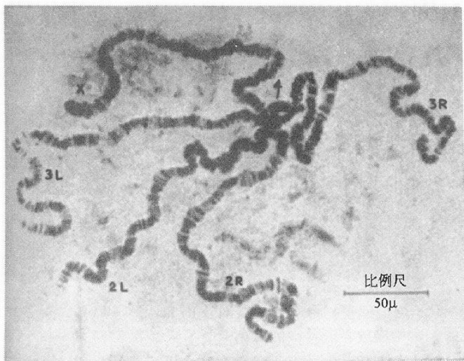
图版V a和b. 果蝇唾液腺体中染色体的显微照片。从图中可以看到倒位和相互易位的现象； c. 雌性果蝇幼体染色体的显微照片。图中标有X的是紧紧挨在一起的一对X染色体。2L和2R是第二对染色体，3L和3R是第三对，标有4的是第四对
