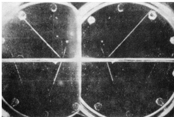
图版 II a. 开始于云室外壁和中央铅片的宇宙线簇射。在磁场的作用下，簇射产生的正、负电子向相反方向偏转。b. 宇宙线粒子在中央隔片上引起核衰变
