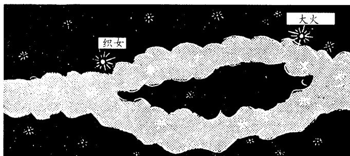
图 112 向银心看去，给人的感觉是这条神话中的河分成两汊
